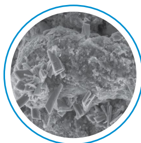
Grânulo de adubo ADP NERGETIC após humedecido e seco. Nutrientes protegidos no gel
